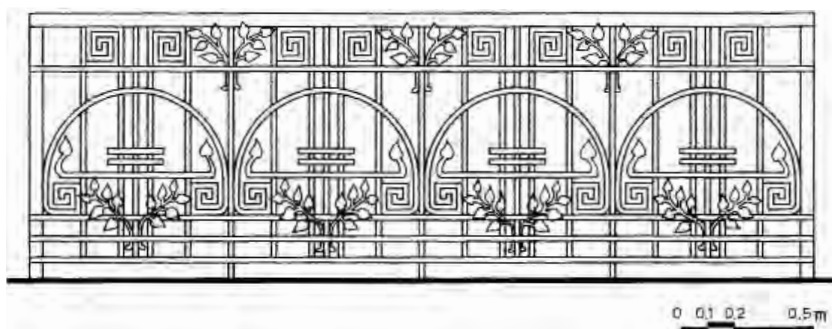
Εικόνα 168. Κυκλίδωμα στην οδό Φανουράκη. Νιοχώρι, Πόλη της Ρόδου.
