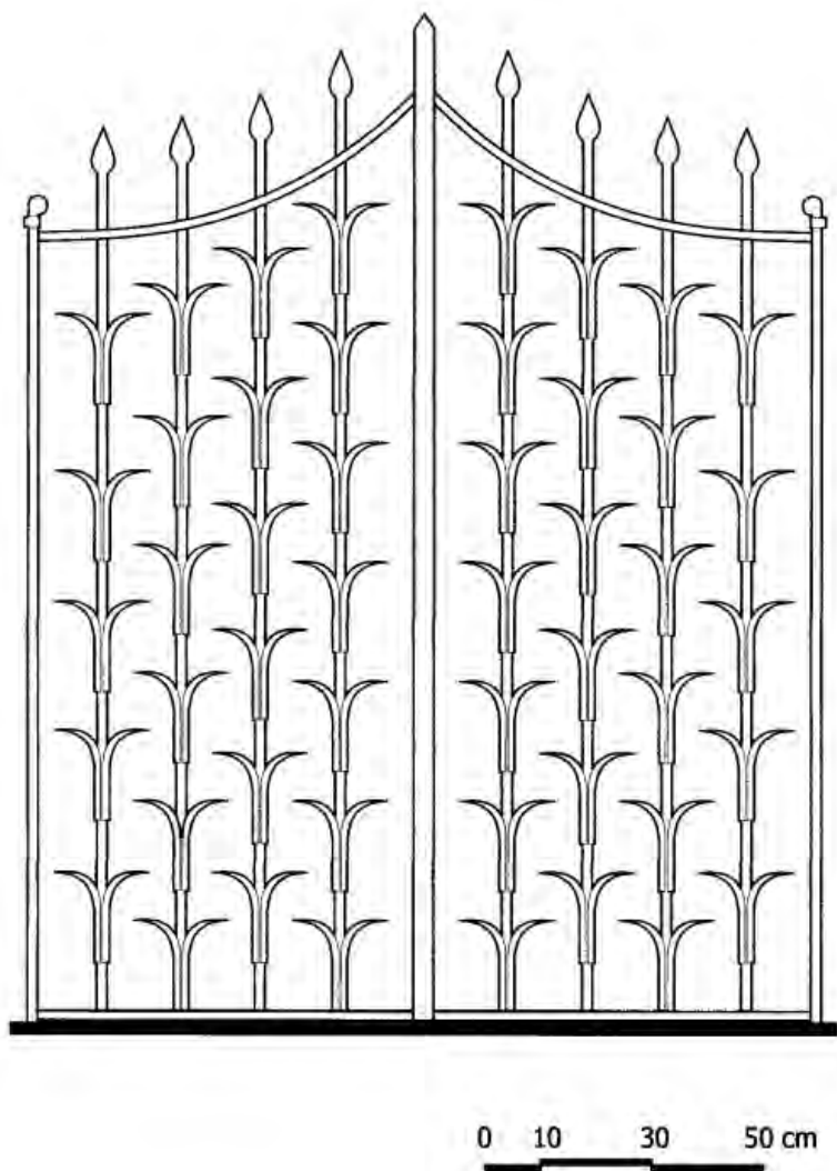
Εικόνα 47. Αύλόθυρα στο Παλαιό Δημοτικό Σχολείο Αρχαγγέλου Ρόδου.
