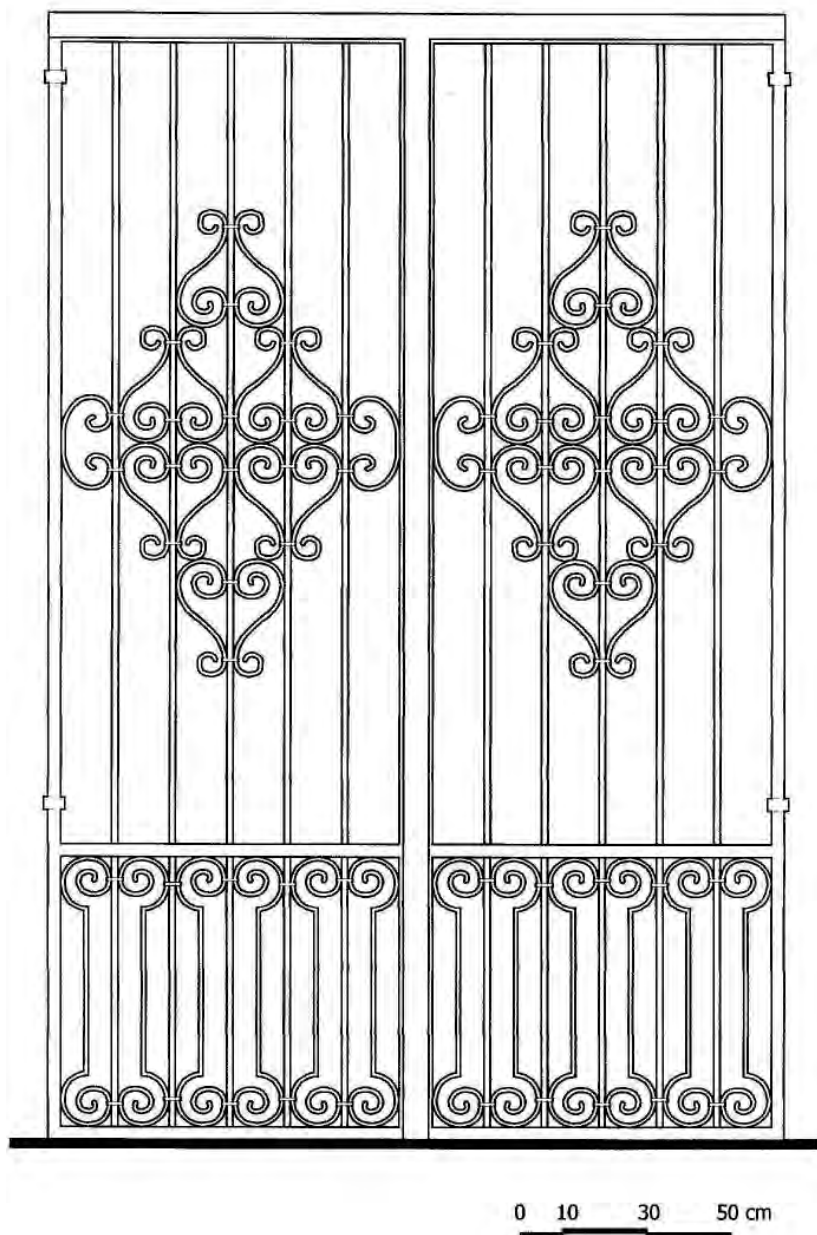
Εικόνα 34. Αύλόθυρα στην οδό Άστρους στην Πόλη της Ρόδου.
