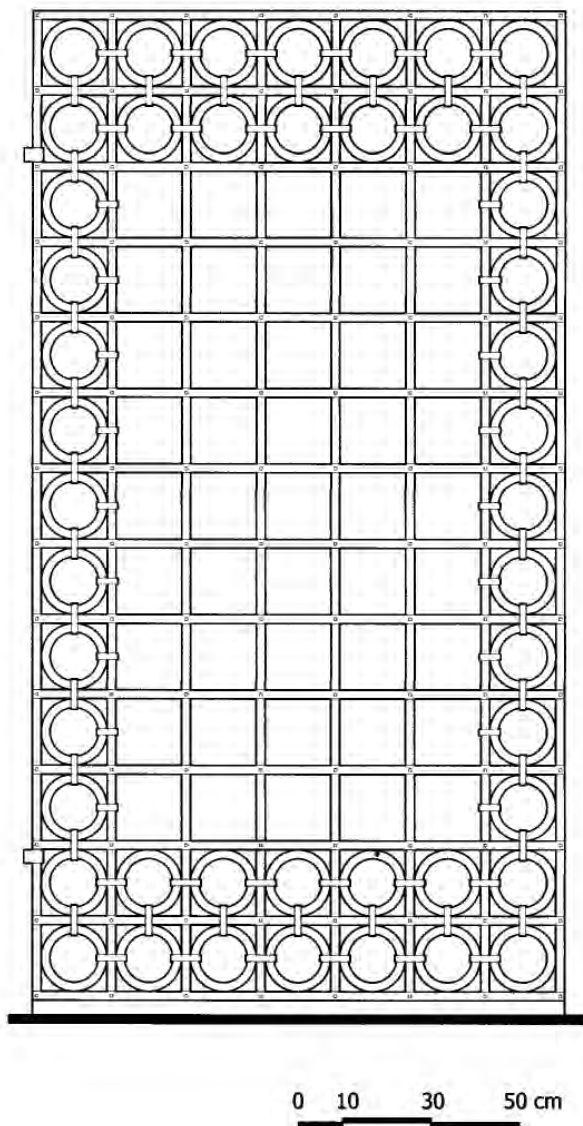
Εικόνα 14. Αύλόθυρα στην οδό Παπαλουκά, στην Πόλη της Ρόδου.
