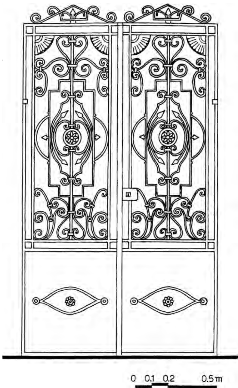
Εικόνα 68. Αύλόθυρα στη Μαλώνα, Ρόδος.
