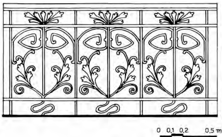
Εικόνα 163. Κιγκλίδωμα στην οδό 25ης Μαρτίου, στην Πόλη της Ρόδου.
