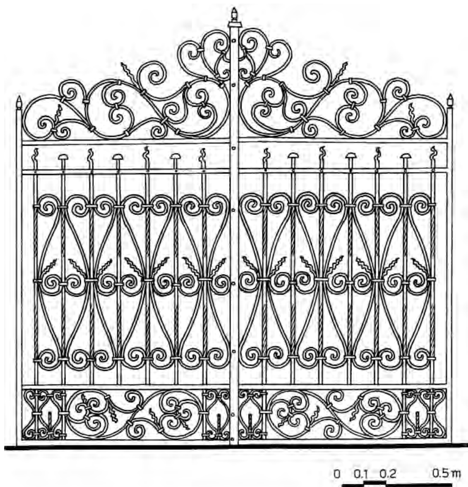
Εικόνα 15. Αυλόθυρα στην πλατεία Κωσταρίδη στην Πόλη της Ρόδου.
