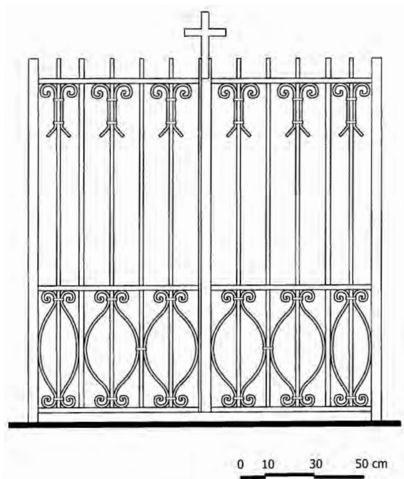
Εικόνα 10. Αύλόθυρα στο Ναό του Αγίου Έλευθερίου στην Πόλη της Ρόδου.
