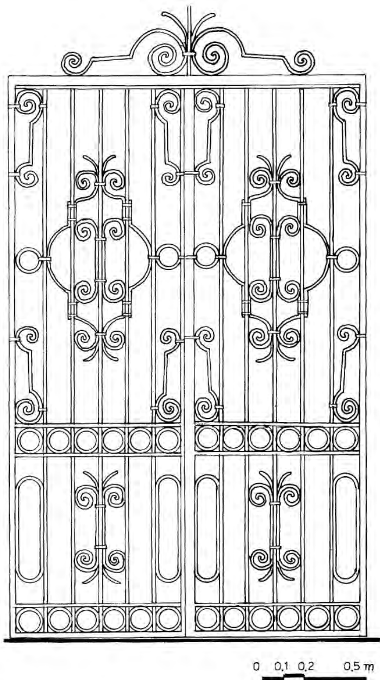
Εικόνα 35. Αυλόθυρα στην οδό Αρχ. Δαμασκηνοῦ, στην Πόλη τῆς Ρόδου.
