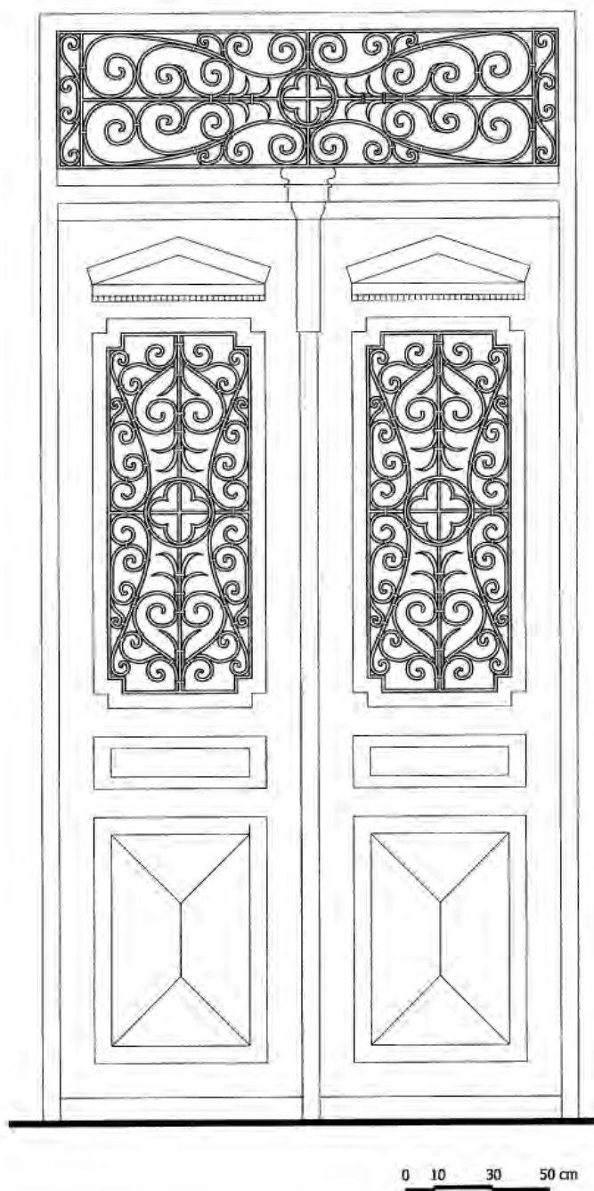
Εικόνα 121. Σιδεριά σέ θύρα οικίας στη Λέρο.
