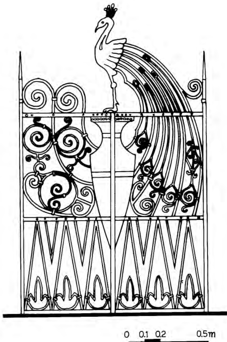
Εικόνα 18. Αυλόθυρα στην Πόλη της Ρόδου.
