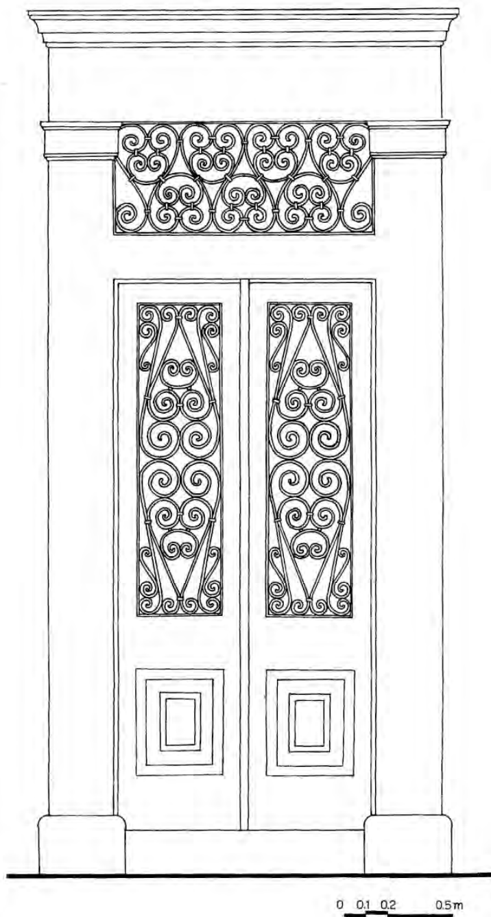
Εικόνα 100. Σιδεριά σέ θύρα οικίας στην Πόλη της Ρόδου.
