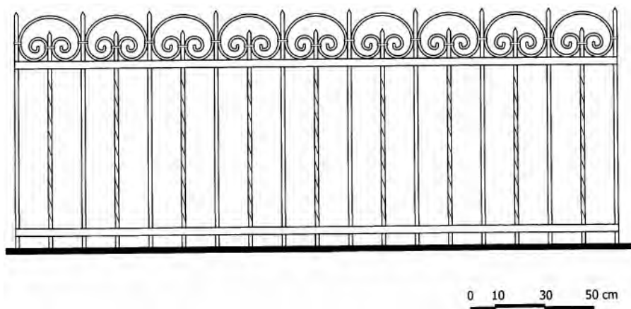
Εικόνα 137. Κιγκλίδωμα στη Πλατεία Κουντουριώτη στη Πόλη της Ρόδου.
