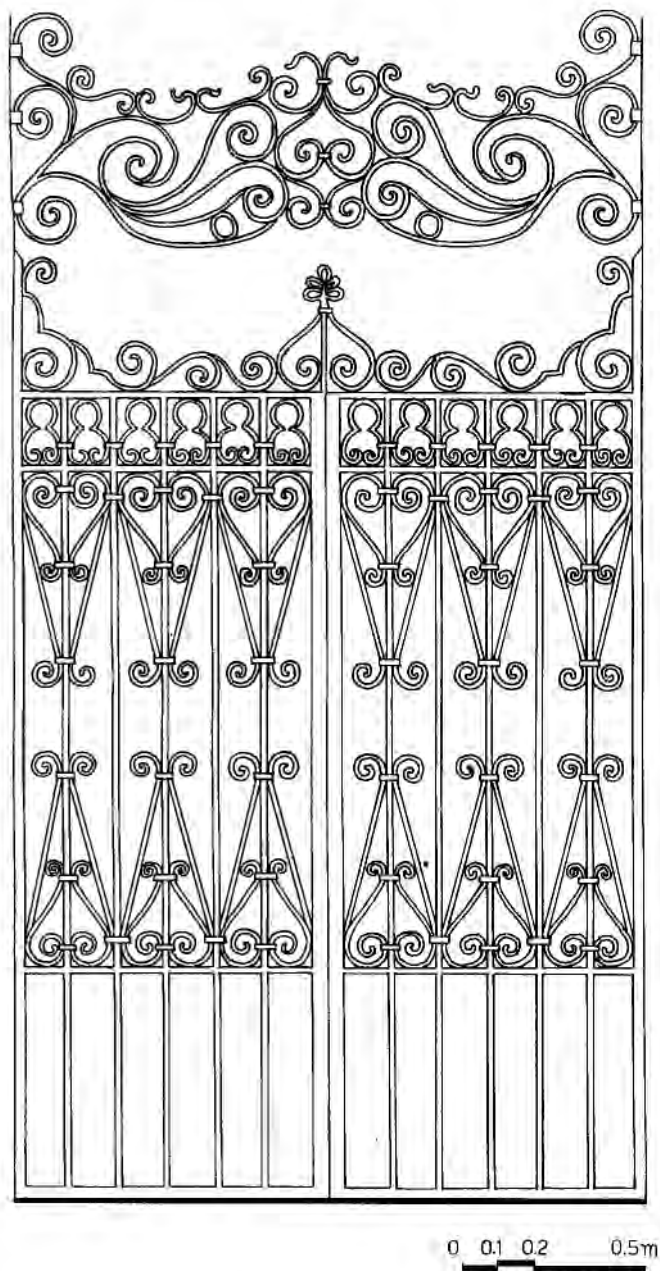
Εικόνα 13. Αύλόθυρα στην οδό Παπαλουκά στην Πόλη της Ρόδου.
