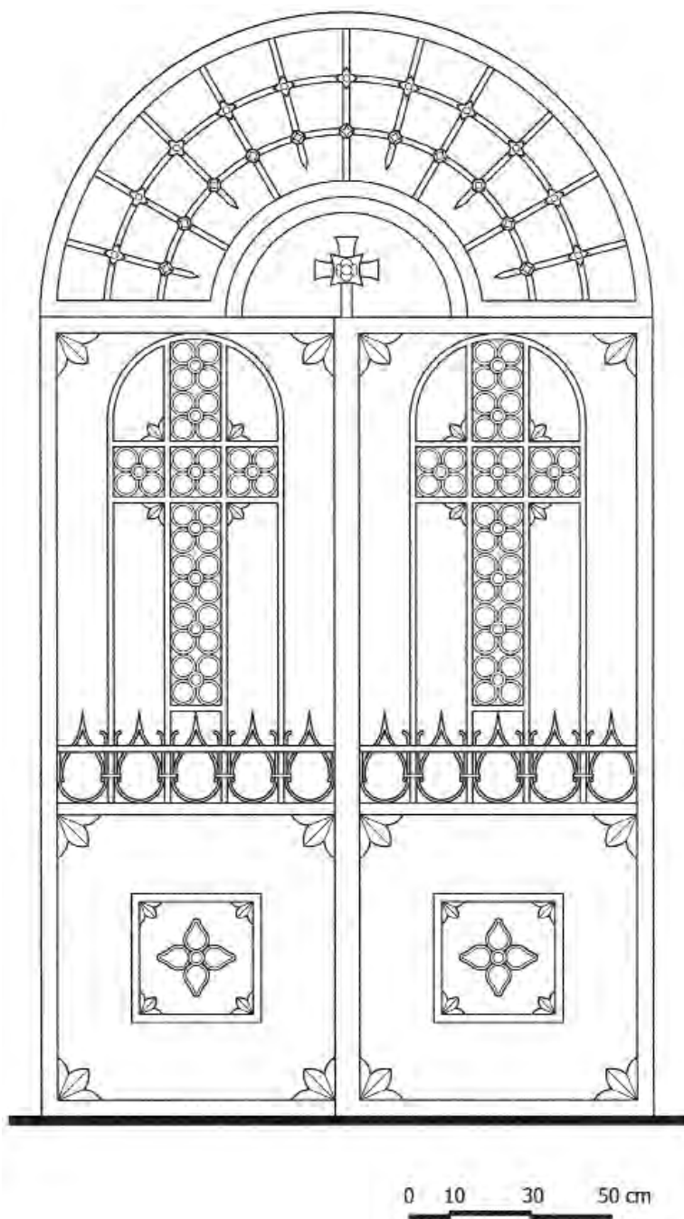
Εικόνα 79. Αύλόθυρα στό Ναό τοῦ Ταξιάρχη Μιχαήλ στήν Λάρδο Ρόδου.
