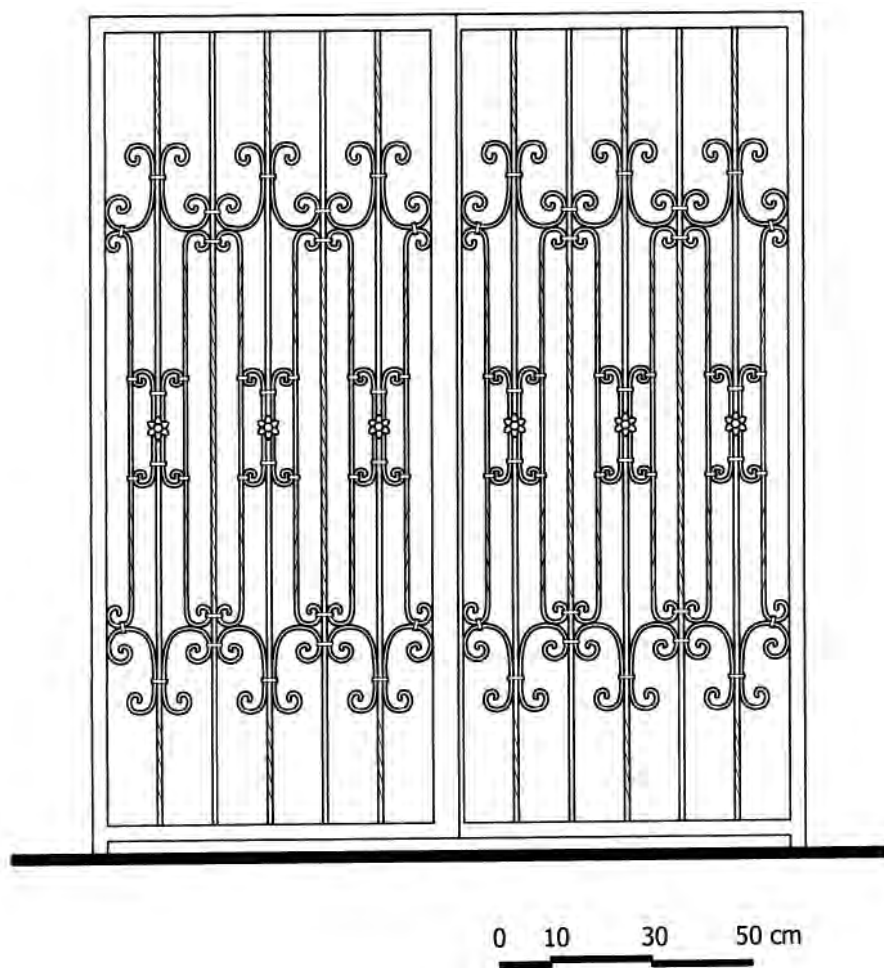
Εικόνα 39. Αυλόθυρα στην οδό Δημητρίου Παππᾶ στην Πόλη της Ρόδου.
