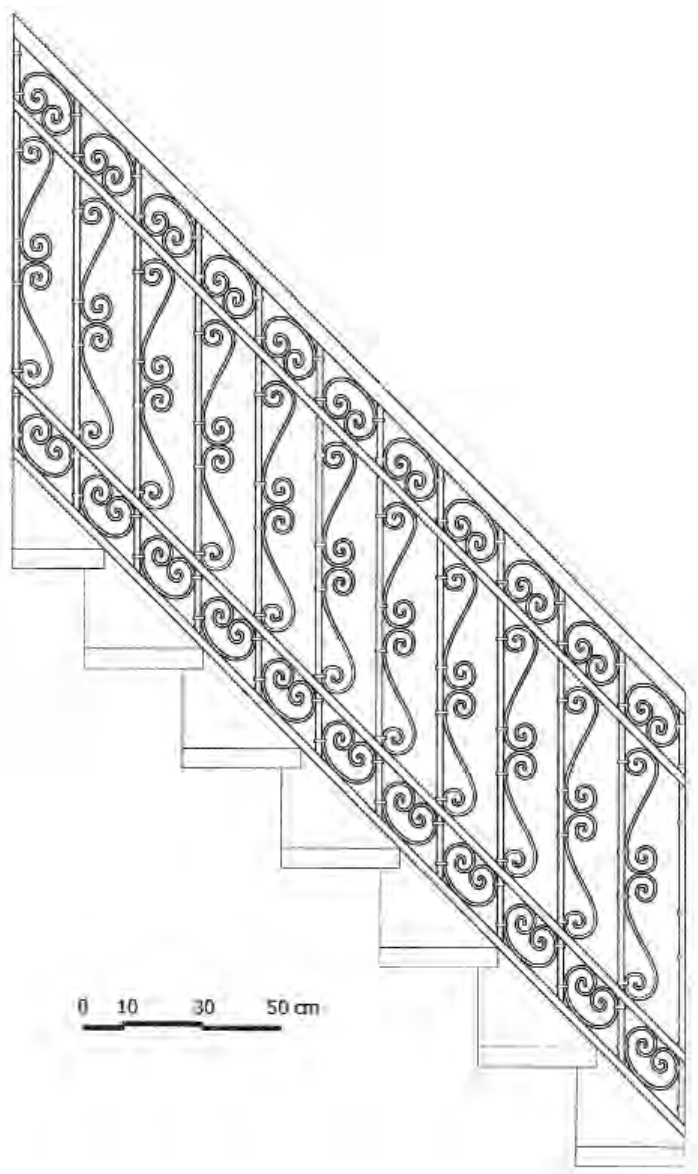
Εικόνα 198. Κιγκλίδωμα στην Έμπωνα Ρόδου.
