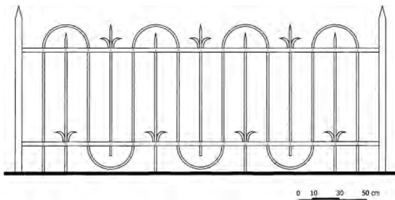
Εικόνα 154. Κιγκλίδωμα στην οδό Στ. Καζούλη, στην Πόλη της Ρόδου.
