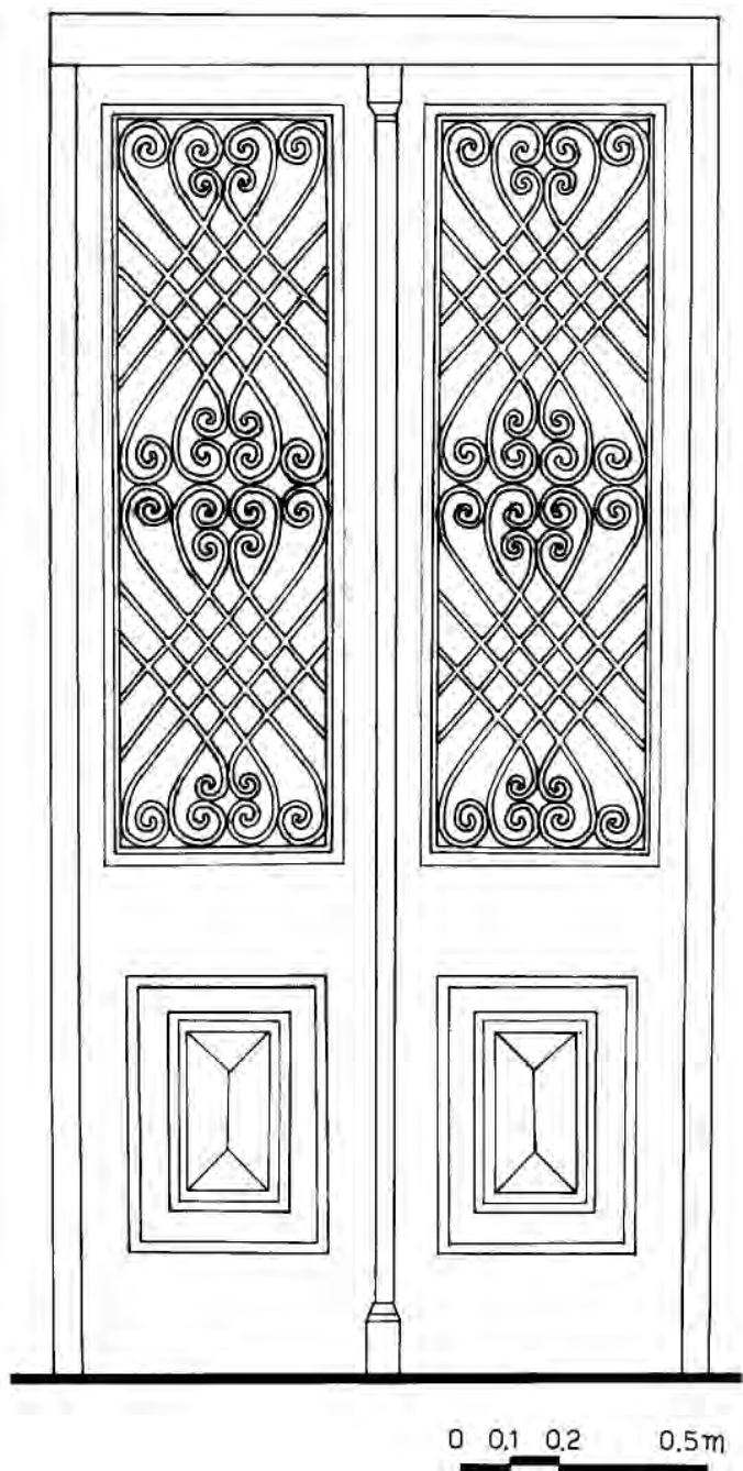
Εικόνα 110. Σιδεριά σέ θύρα οίκιας στήν Πόλη τῆς Ρόδου.
