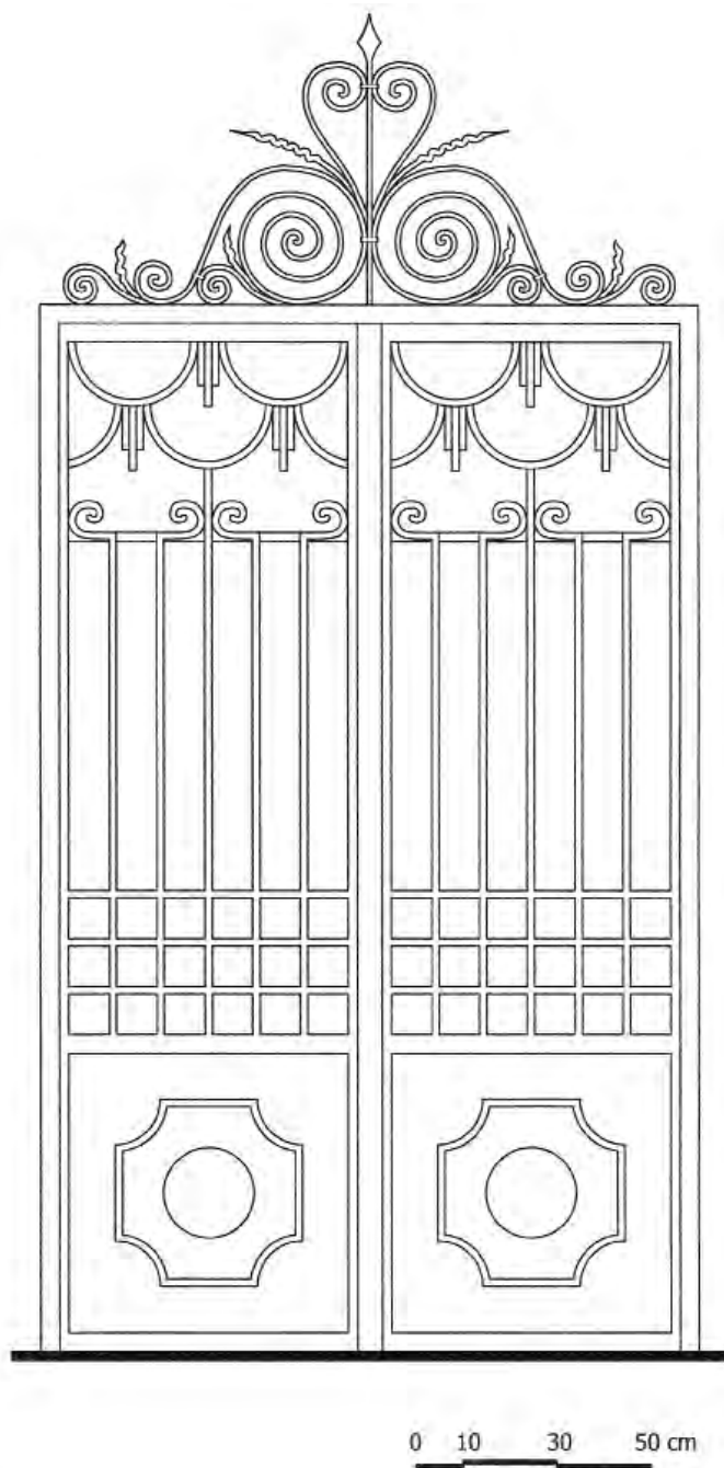
Εικόνα 12. Αύλόθυρα στην οδό Στρατηγού Ζήση, στην Πόλη της Ρόδου.
