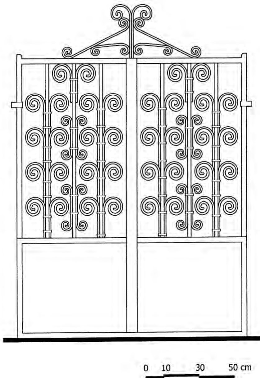
Εικόνα 37. Αυλόθυρα στην οδό Έρνεστ Μπεβίν στην Πόλη της Ρόδου.
