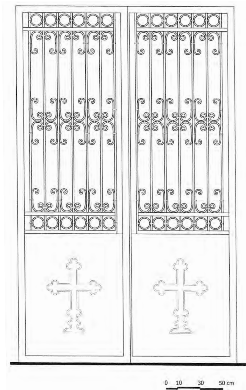
Εικόνα 4. Αυλόθυρα στο Ναό του Αγίου Ιωάννου στην Πόλη της Ρόδου.
