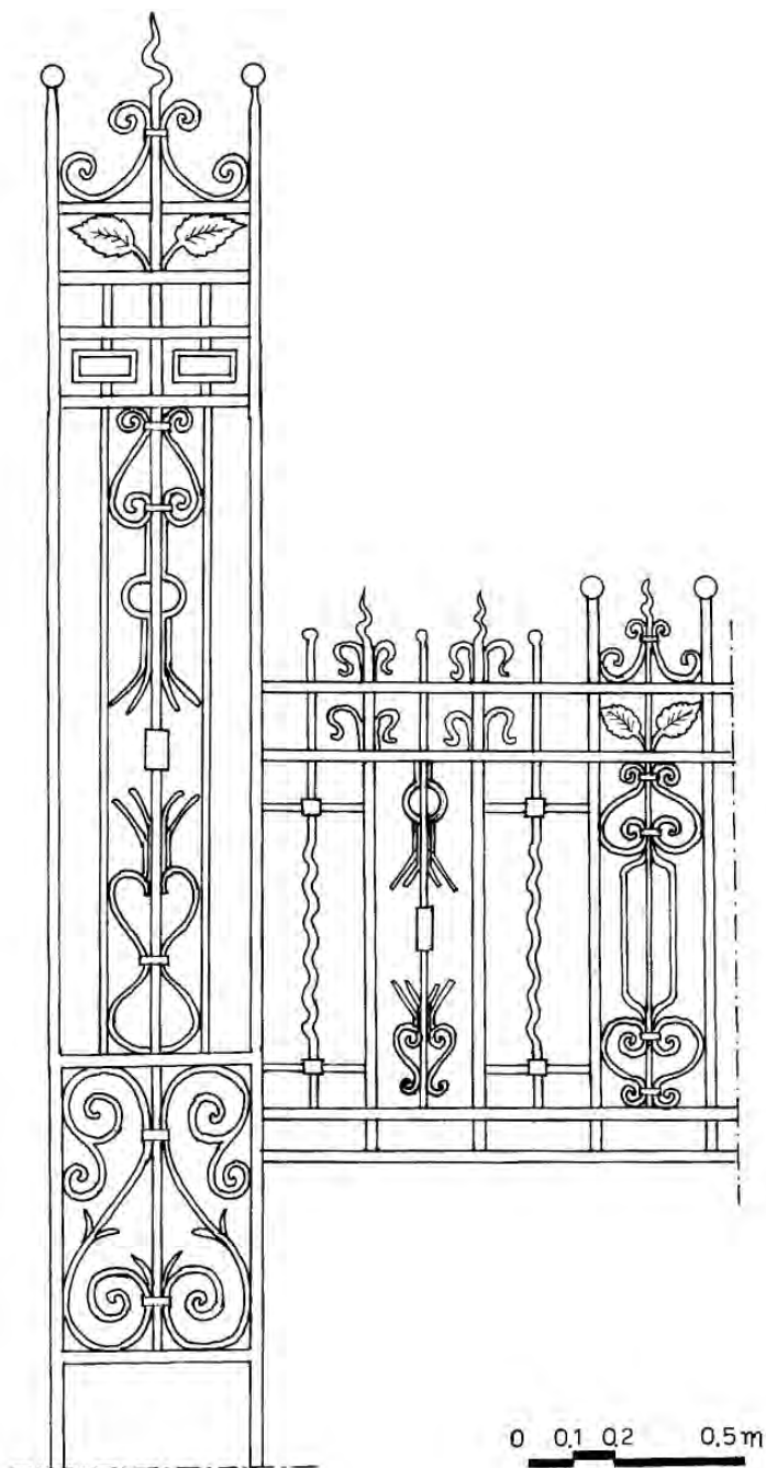
Εικόνα 150. Κυκλίδωμα στην οδό Χιμάρας, στην Πόλη της Ρόδου.
