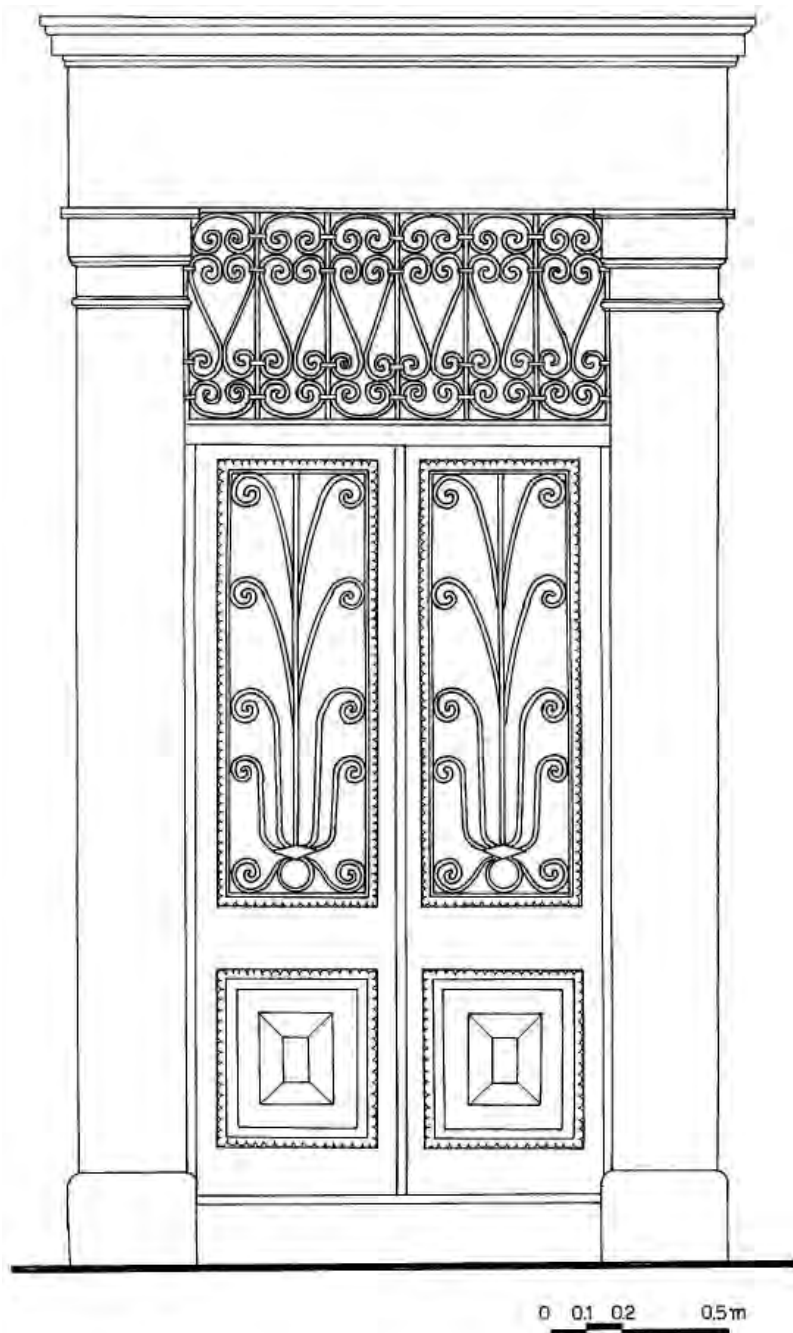
Εικόνα 94. Σιδεριά σέ θύρα οικίας στην Πόλη της Ρόδου.
