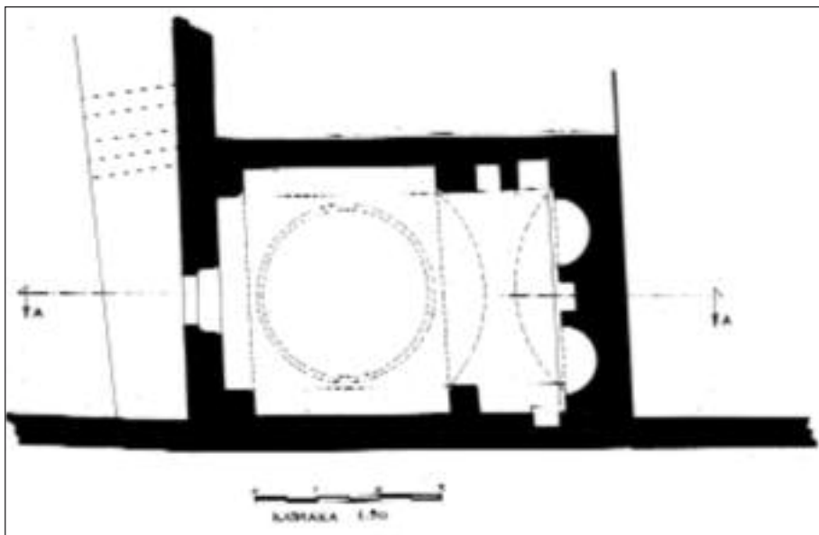
Εικ. 46 ΠΑΤΜΟΣ: ΑΓΙΟΣ ΑΘΑΝΑΣΙΟΣ ΣΤΗ ΧΩΡΑ ΚΑΤΟΨΗ
