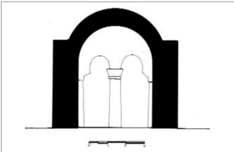
Εικ. 28 ΚΑΡΠΑΘΟΣ ΑΡΚΑΣΑ - ΑΓΙΟΣ ΝΙΚΟΛΑΟΣ ΤΟΜΗ
