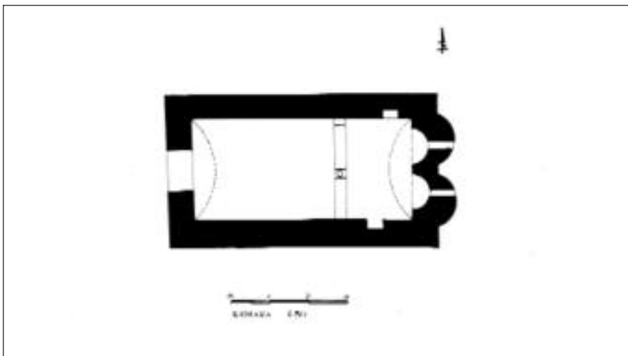
Εικ. 33 ΚΑΡΠΑΘΟΣ: ΜΕΣΟΧΩΡΙ ΑΓΙΟΣ ΓΕΩΡΓΙΟΣ ΤΟΥ ΒΟΥΝΟΥ ΚΑΤΩΨΗ
