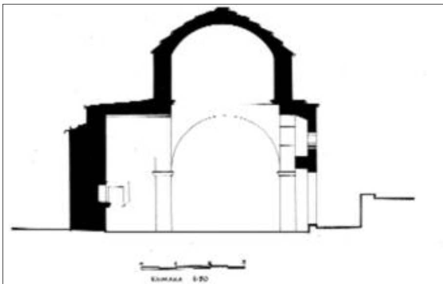
Εικ. 47 ΠΑΤΜΟΣ: ΑΓΙΟΣ ΑΘΑΝΑΣΙΟΣ ΣΤΗ ΧΩΡΑ ΤΟΜΗ Α-Α'
