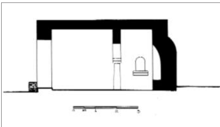
Εικ. 27 ΚΑΡΠΑΘΟΣ ΑΡΚΑΣΑ - ΑΓΙΟΣ ΝΙΚΟΛΑΟΣ ΤΟΜΗ
