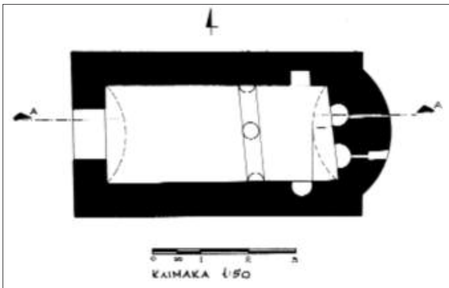
Εικ. 26 ΚΑΡΠΑΘΟΣ ΑΡΚΑΣΑ - ΑΓΙΟΣ ΝΙΚΟΛΑΟΣ ΚΑΤΟΨΗ
