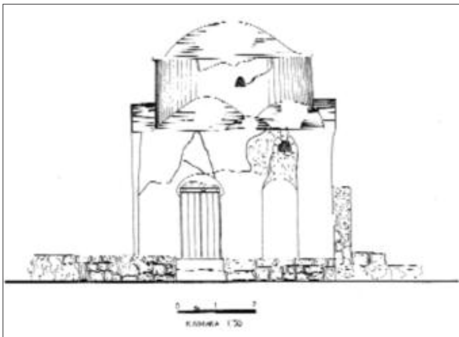
Εικ. 39 ΚΑΡΠΑΘΟΣ: ΜΕΣΟΧΩΡΙ - ΛΕΥΚΟ ΑΓΙΟΣ ΓΕΩΡΓΙΟΣ ΟΥΗ
