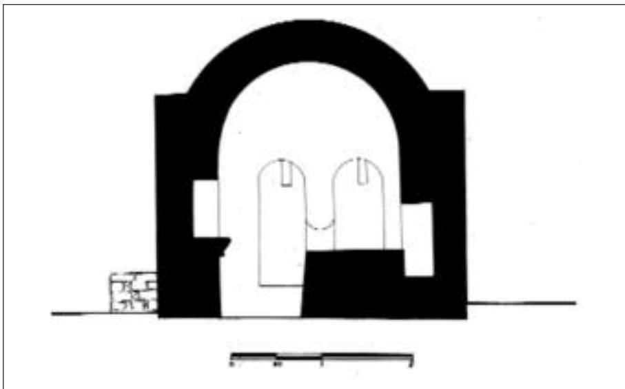
Εικ. 29 ΚΑΡΠΑΘΟΣ ΑΡΚΑΣΑ - ΑΓΙΟΣ ΝΙΚΟΛΑΟΣ ΤΟΜΗ
