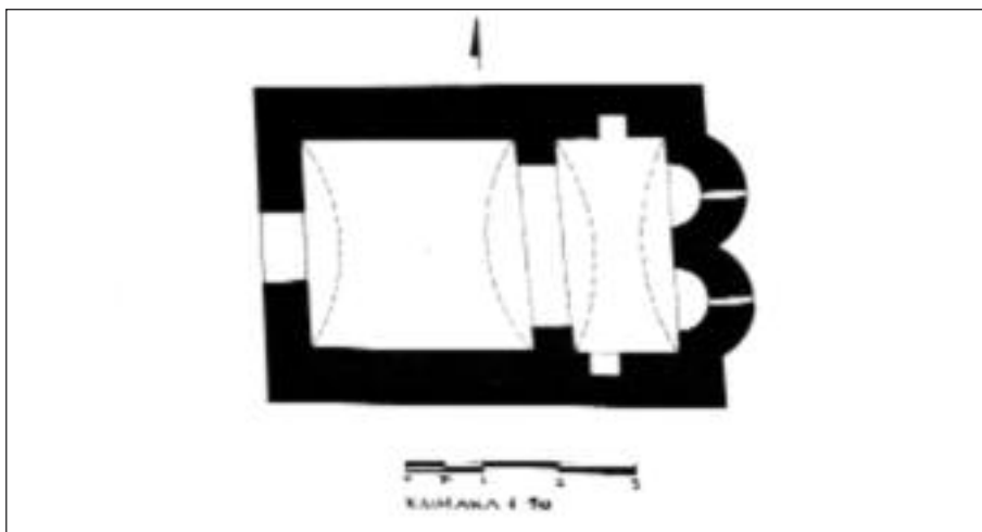
Εικ. 40 ΚΑΡΠΑΘΟΣ: ΟΘΩΣ - ΣΤΕΣ ΑΓΙΟΙ ΓΕΩΡΓΙΟΣ ΓΕΩΡΓΙΟΣ ΚΑΙ ΔΗΜΗΤΡΙΟΣ ΚΑΤΟΥΗ
