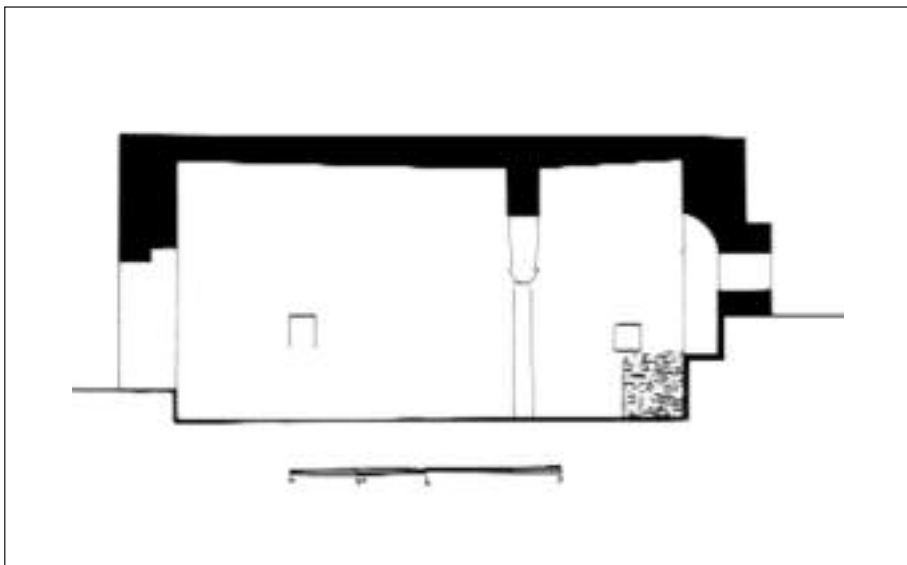
Εικ. 34 ΚΑΡΠΑΘΟΣ: ΜΕΣΟΧΩΡΙ ΑΓΙΟΣ ΓΕΩΡΓΙΟΣ ΤΟΥ ΒΟΥΝΟΥ ΤΟΜΗ
