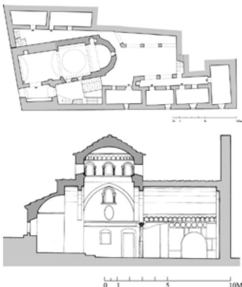
4. Κάτοψη και κατά μήκος τομή (άποτύπωση Μ. Σάνδαλος, ηλεκτρονική επεξεργασία Γ. Σταυρόπουλος).
