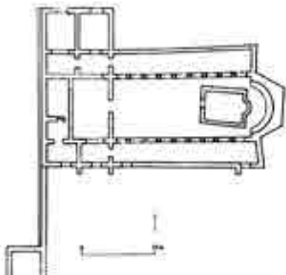
A. Κάτοψη παλαιοχριστιανικής βασιλικής Ἀγίας Ἀναστασίας. Ἀπολλακιά-Ρόδος. Deligiannakis, 2016, 134, fig. 76 Rhodes 60.
