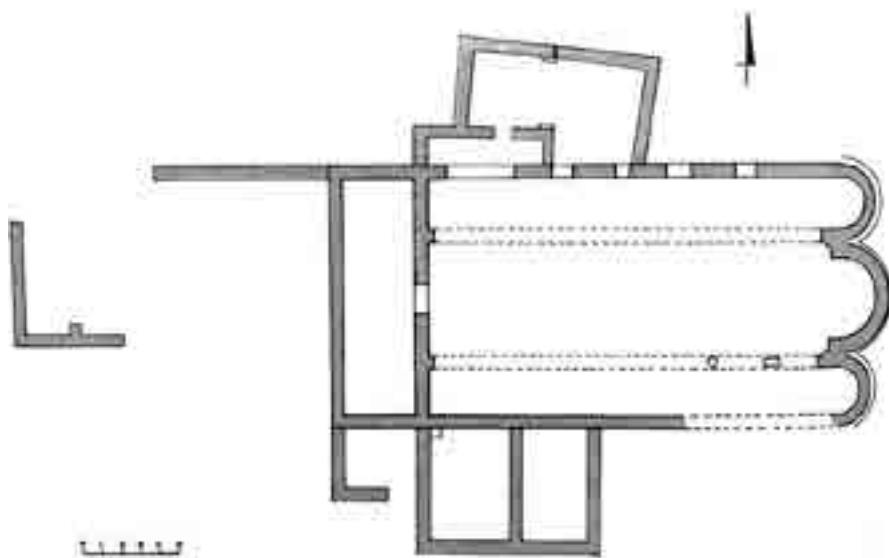
Β. Κάτοψη παλαιοχριστιανικής βασιλικής Παλαιάς Παναγιάς - Τέλενδος. Karabatsos, 1994, 306, fig. 18.
