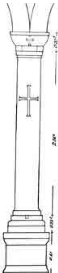
Α. Σχεδιαστική αναπαράσταση ενός από τα στηρίγματα των κιονοστοιχιών της βασιλικής Μαστιχάρι, Κως. Όρλάνδος, 1966, εικ. 14.
