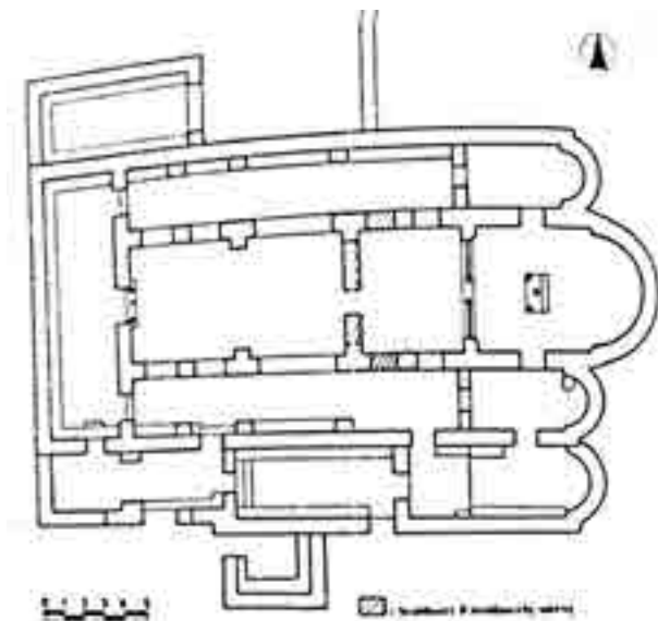
Α. Κάτοψη παλαιοχριστιανικής βασιλικής Χοχλακάς - Τέλενδος. Κουτελλάς, 1998, 1008, εικ. 12.
