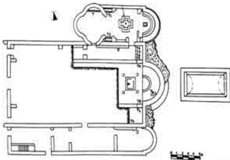
Α. Κάτοψη παλαιοχριστιανικής βασιλικής. Παλαιοπαναγία. Κάλυμνος-Άγιος Παντελεήμων. Deligiannakis, 2016, 323, fig. 26.
