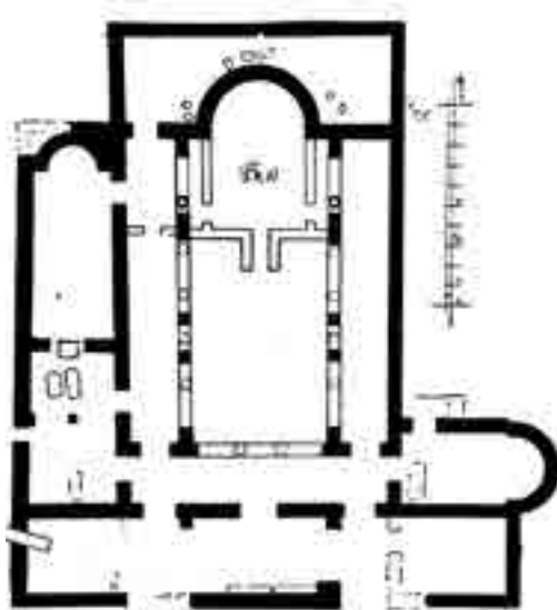
Α. Κάτοψη βασιλικής Τούμπας στη Θεσσαλονίκη. Σωτηρίου, 1929, εικ. 9.
