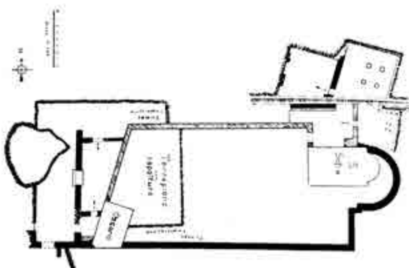
Α. Κάτοψη παλαιοχριστιανικής βασιλικής Ἀγίας Ἀναστασίας. Κάρπαθος-Ἀρκάσα. Σωτηρίου, 1929, 196, εἰκ.29.
