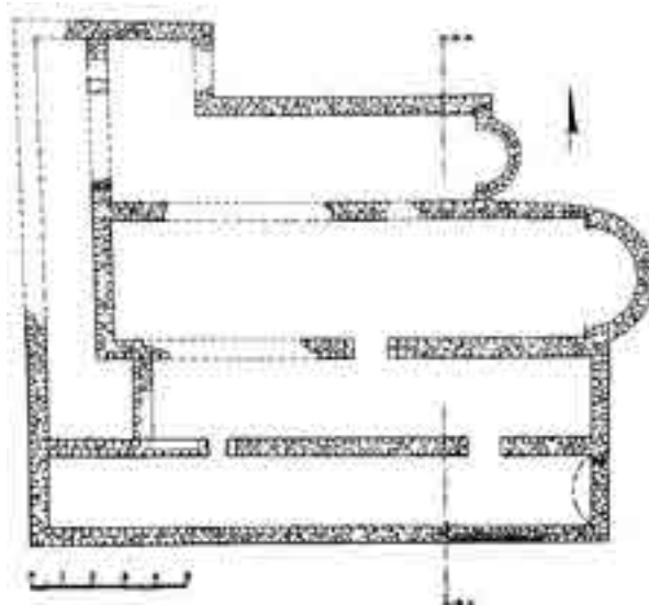
Α. Κάτοψη παλαιοχριστιανικής βασιλικής. Ἀνατολική Ἐκκλησία. Κάλυμνος. Karabatsos, 1994, 348, fig. 39.
