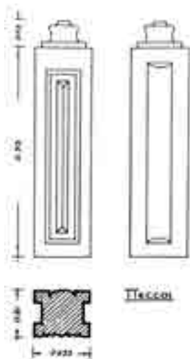
Α. Σχεδιαστική απεικόνιση πεσσίσκου από βασιλική Λέσβου. Όρλάνδος, 1929, εικ. 19.
