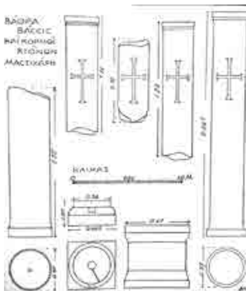
Α. Σχεδιαστική αναπαράσταση: βάθρο, βάσεις και κορμοί κίωνων τῆς βασιλικῆς στό Μαστιχάρι, Κῶς. Όρλάνδος, 1966, εἰκ. 10.
