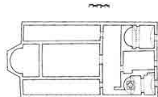
Γ. Κάτοψη παλαιοχριστιανικής βασιλικής. Κολύμπια-Ρόδος. Βολανάκης, 1984, 693, σχ. 1.
