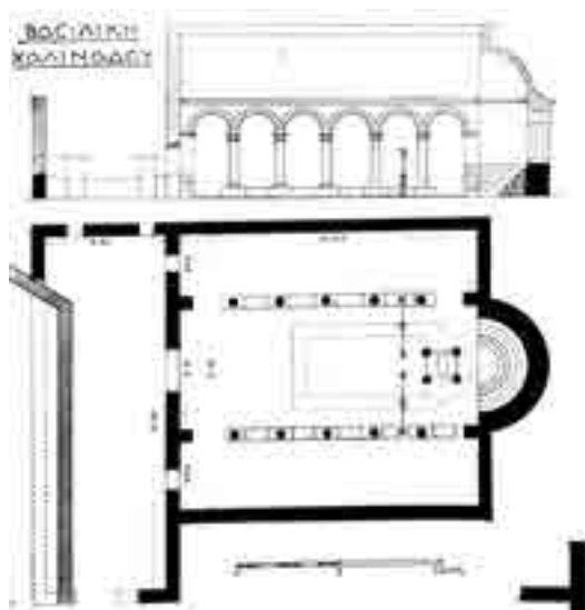
Κάτοψη καί κατά μήκος τής βασιλικής τοῦ Χαλινάδου Λέσβου. Ὁρλάνδος, 1937, εἰκ.2.
