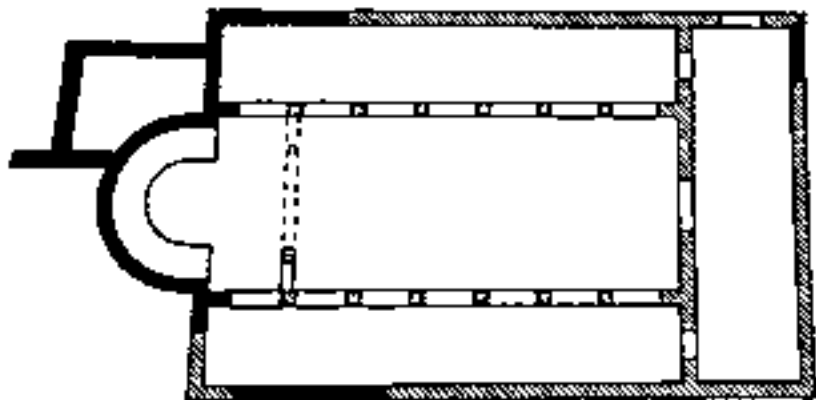
Α. Κάτοψη παλαιοχριστιανικής βασιλικής τῆς Ἀντιμάχειας. Κῶς. Ὅρλάνδος, 1966, 102, εἰκ. 102.
