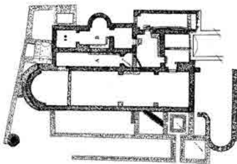
Α. Κάτοψη παλαιοχριστιανικής βασιλικής στο Παρθένι της Λέρου. Μιχαηλίδου, 1993, 43, σχ. ΙΙΙ.
