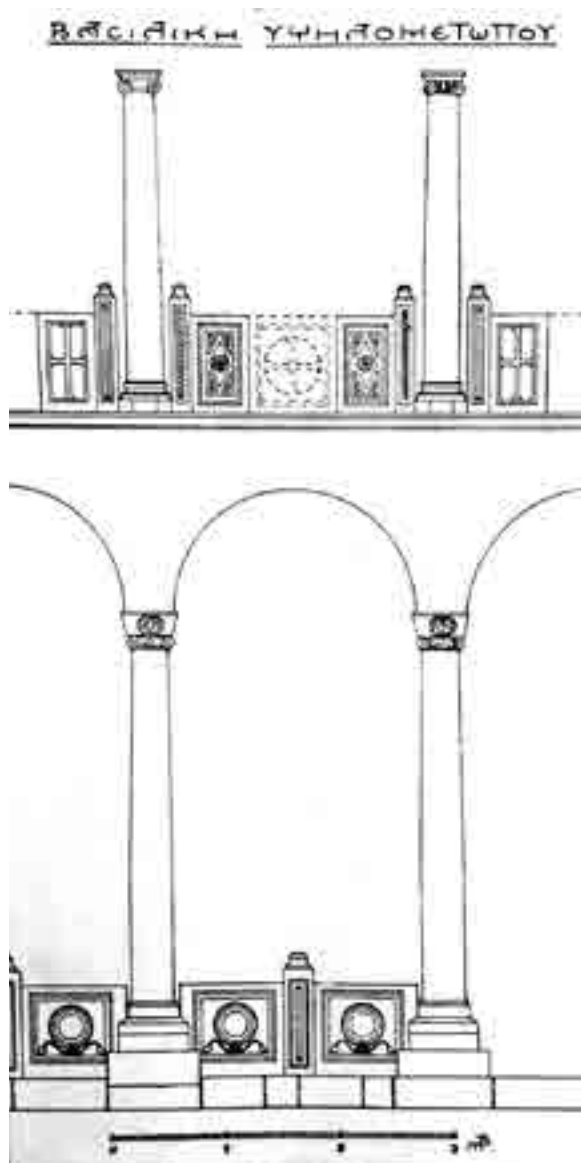
Ἀναπαράσταση τμήματος τῶν κιονοστοιχιῶν τῆς βασιλικῆς Ὑψηλομετώπου Λέσβου. Ὅρλάνδος, 1929, εἰκ. 18.
