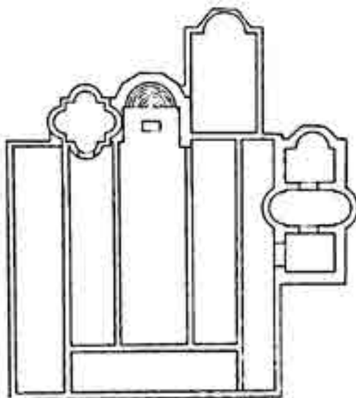
Α. Κάτοψη παλαιοχριστιανικής βασιλικής Α', Ἀρνίθα - Ρόδος. Βολανάκης, 1979, 269, εικ. 1.
