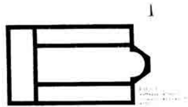
Α. Κάτοψη παλαιοχριστιανικής βασιλικής Α΄. Βρυκούς-Κάρπαθος. Βολανάκης, 1998, 229.
