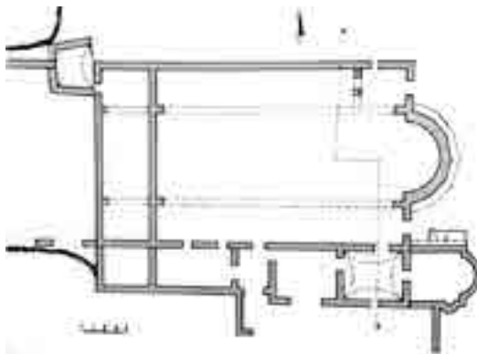
Α. Κάτοψη παλαιοχριστιανικής βασιλικής Αγίου Βασιλείου. Τέλενδος. Karabatsos, 1994, 298, fig. 14.
