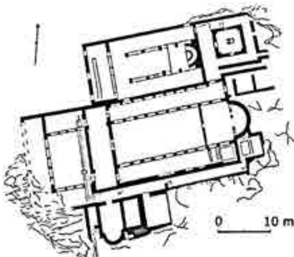
Α. Κάτοψη παλαιοχριστιανικής βασιλικής Α' (μεγάλη) Άγιος Στέφανος. Κώς. Deligiannakis, 2016, 158, fig.110. Kos 2.2.
