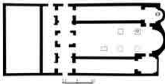
Γ. Κάτοψη παλαιοχριστιανικής βασιλικής. Κάλαθος-Ρόδος. Deligiannakis, 2016, 134, fig. 74, Rhodes 53.
