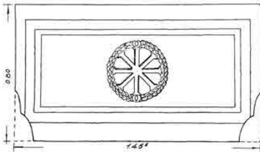
Β. Σχεδιαστική απεικόνιση θωρακίου από τη βασιλική Ύψηλομετώπου Λέσβου. Όρλάνδος, 1929, εικ. 25.
